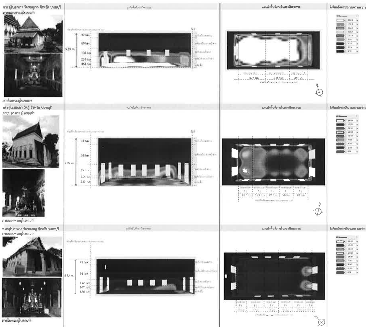
ภาพที่ 12 ข้อมูลผลค่าปริมาณความสว่างของพระอุโบสถเพื่อทดสอบคุณลักษณะของแสงต่อพื้นที่ ที่มา: ผู้วิจัย
