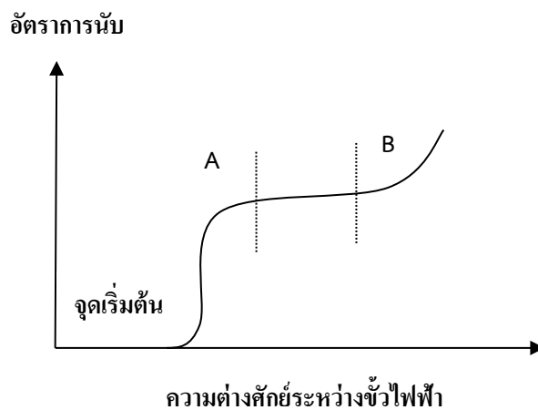
ภาพที่ 2 กราฟแสดงคุณสมบัติของหัววัดไกเกอร์-มูลเลอร์
