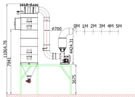
ภาพที่ 1 จุดที่ทำการวัดความเร็วลมจากปลายปล่องลมทิ้งของเครื่องดูดฝุ่นชนิดถุงกรอง ขนาด 50 แรงม้า
