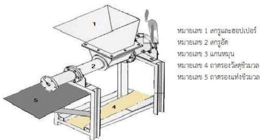
รูปที่ 1 เครื่องอัดแท่งชีวมวลแบบมือหมุน
