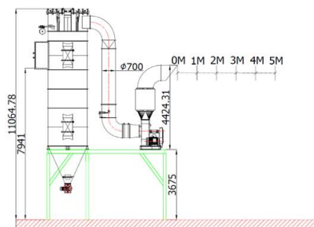
ภาพที่ 1 จุดที่ทำการวัดความเร็วลมจากปลายปล่องลมทิ้งของเครื่องดูดฝุ่นชนิดถุงกรอง ขนาด 50 แรงม้า
