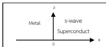
ภาพที่ 1 แบบจำลองรอยต่อระหว่าง โลหะ/สารตัวนำยิ่งยวด
