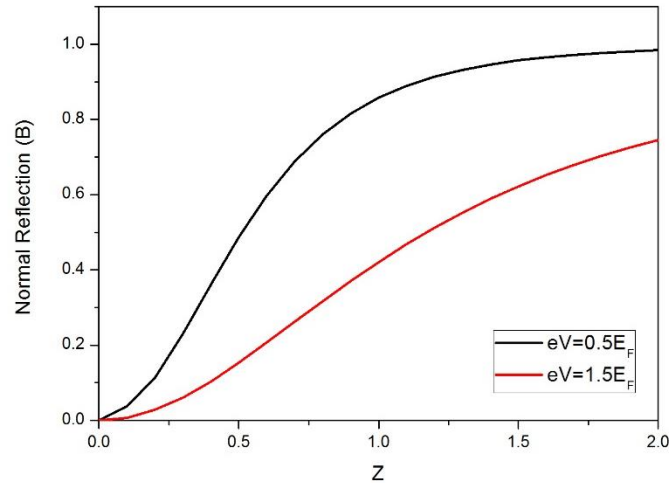
ภาพที่ 3 โอกาสของการสะท้อนกลับของอิเล็กตรอนที่เป็นฟังก์ชันของกัมพางค์กัฏระหว่าง eV = 0.5E_F และ eV = 1.5E_F
