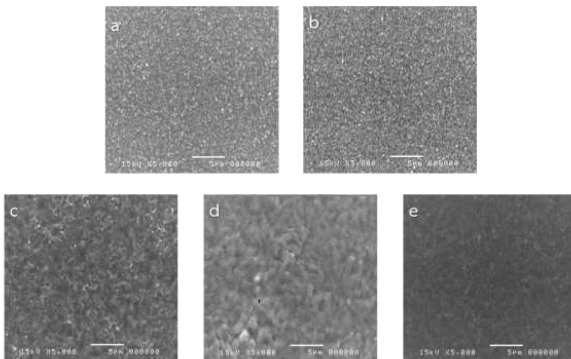
ภาพที่ 4 ลักษณะพื้นผิวและผลึกของ a) फिल्म PEDOT:PSS b) फिल्म \text{Cu}_2\text{O} c) फिल्मเพอรอฟสไกต์ที่สร้างบนฟิล์ม PEDOT:PSS d) फिल्मเพอรอฟสไกต์ที่สร้างบนฟิล์ม \text{Cu}_2\text{O} (CuI 5 mg/ml) และ e) फिल्मเพอรอฟสไกต์ที่สร้างบนฟิล์ม PEDOT:PSS/ฟิล์ม \text{Cu}_2\text{O} (CuI 5mg/ml)
