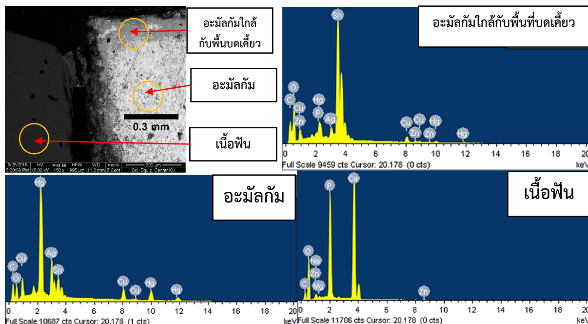
ภาพที่ 5 ผลการวิเคราะห์จากกล้องจุลทรรศน์อิเล็กตรอนแบบส่องกราด แสดงสัญญาณและสเปกตรัมแสดงปริมาณแต่ละธาตุของตัวอย่างฟันตัวอย่างที่ 12 วงกลมสีแดงแสดงพื้นที่วิเคราะห์ใกล้กับส่วนที่ใช้สำหรับการบัดเคียว (Area 1) พื้นที่ที่เป็นอะมัลกัมตรงกลางชิ้นตัวอย่าง (Area 2) และส่วนที่เป็นเนื้อฟัน (Area 3)
