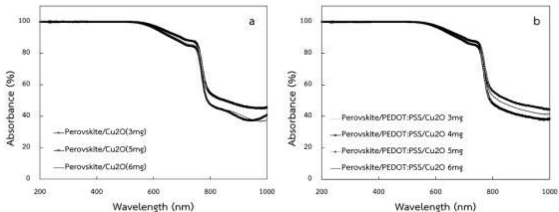
ภาพที่ 3 ประสิทธิภาพการดูดกลืนแสงของชั้นฟิล์มเพอรอฟสไกต์ที่สร้างบนวัสดุนำโพลีเมอร์ต่างกัน
