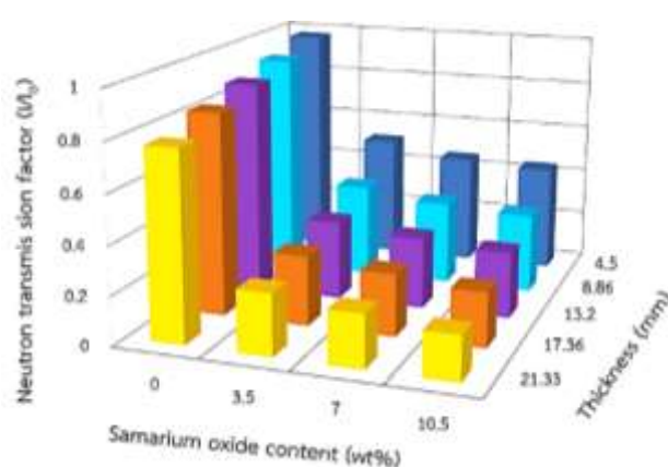
ภาพที่ 5 ค่าการลดทอนอนุภาคนิวตรอน ( I/I_0 ) ที่ปรับเปลี่ยนสารตัวเติม Sm 2 O 3 และความหนาของวัสดุเชิงประกอบ
