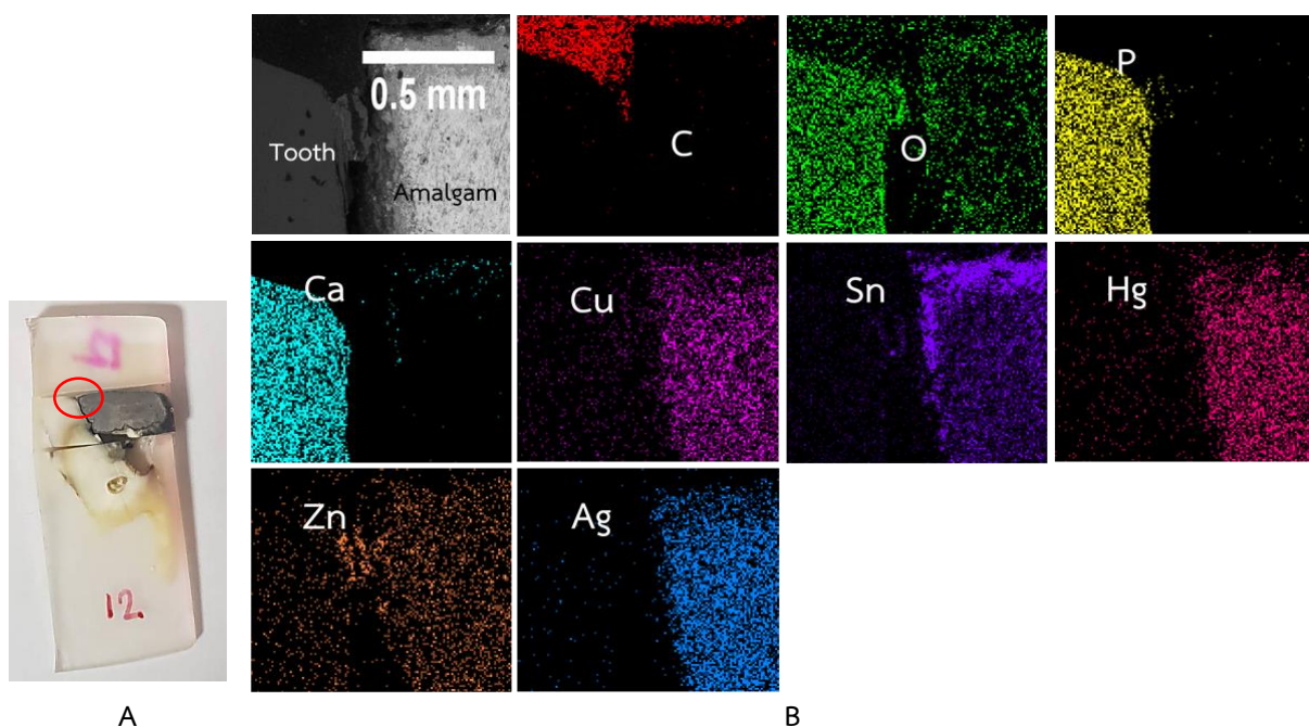
ภาพที่ 4 (A) ภาพตัวอย่างฟันตัดขวางแสดงส่วนที่เป็นอะมัลกัม รอยต่อระหว่างอะมัลกัมและเนื้อฟัน และส่วนที่เป็นเนื้อฟัน วงกลมสีแดง แสดงบริเวณอะมัลกัมที่ใช้ในการวิเคราะห์ด้วยกล้องจุลทรรศน์อิเล็กตรอนแบบส่องกราด (B) ผลการวิเคราะห์จากกล้องจุลทรรศน์อิเล็กตรอนแบบส่องกราด แสดงการกระจายตัวของตัวอย่างฟันตัวอย่างที่ 12
