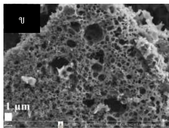
ภาพที่ 2 แสดงลักษณะทางกายภาพที่กล้องขยาย 5000 เท่าของเปลือกกล้วยน้ำหว้าที่เตรียมถ่านกัมมันต์โดยวิธีคาร์บอนเซชันและวิธีกระตุ้นทางเคมี เปรียบเทียบที่ 700°C เป็นเวลา 2 วิธีคาร์บอนเซชัน สเกลบาร์ (ก) ขั้วโม่ง โดย 2 ไมโครเมตร 1 วิธีกระตุ้นทางเคมี สเกลบาร์ (ข) ไมโครเมตร
