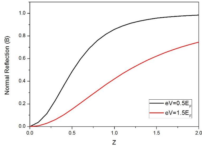
ภาพที่ 3 โอกาสของการสะท้อนกลับของอิเล็กตรอนที่เป็นฟังก์ชันของกัมพาคักยระหว่าง eV = 0.5E_F และ eV = 1.5E_F
