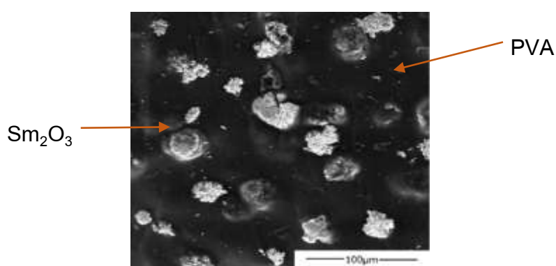
ภาพที่ 4 ลักษณะสัณฐานวิทยาของวัสดุเชิงประกอบ PVA/Sm 2 O 3 ด้วยเทคนิค SEM
