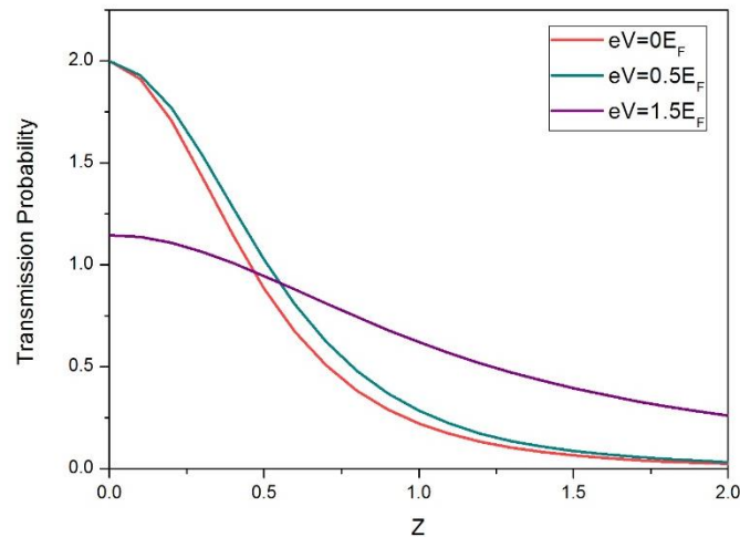
ภาพที่ 4 โอกาสของการทะลุผ่านของอนุภาคที่เป็นฟังก์ชันของกัมพาคักยที่พลังงาน eV = 0E_F , eV = 0.5E_F และ eV = 1.5E_F
